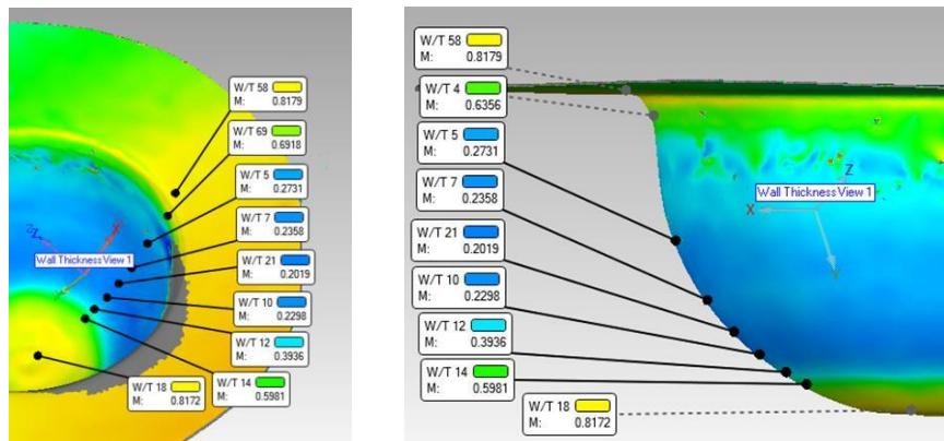
Gambar 15: Distribusi ketebalan dinding produk pada model uji 2.
